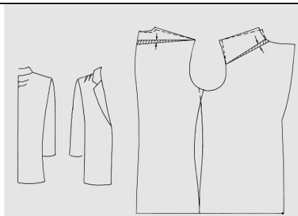
Рис. 31. Наклонные складки по плечевому шву, идущие от среднего шва спинки
